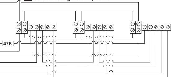
Figure 2 EN: Multiple Unit Connection Procedure FR: Procédure Pour Connecter Plusieurs Appareils ES: Procedimiento para la Conexión de Varias Unidades IT: Schema di collegamento di più unità
