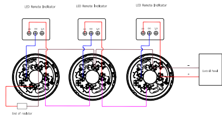
Figure3-2 Wiring
